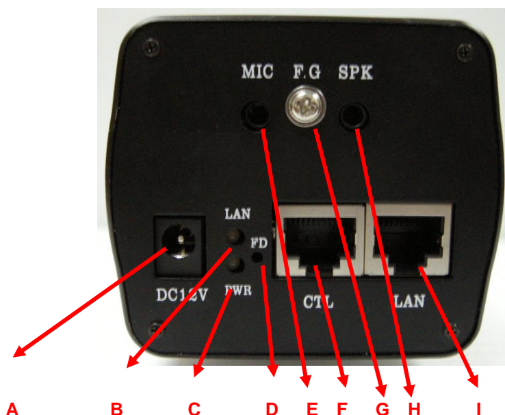
Рисунок 3. Вид сзади MDC-i4260C
